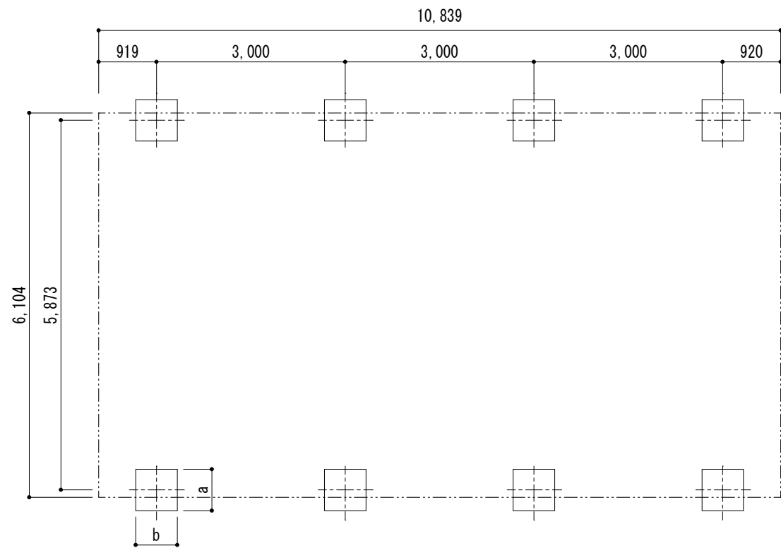
■基礎配置図
